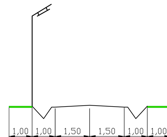
Поперечный профиль лыжни "Тропа Здоровья" А-А
